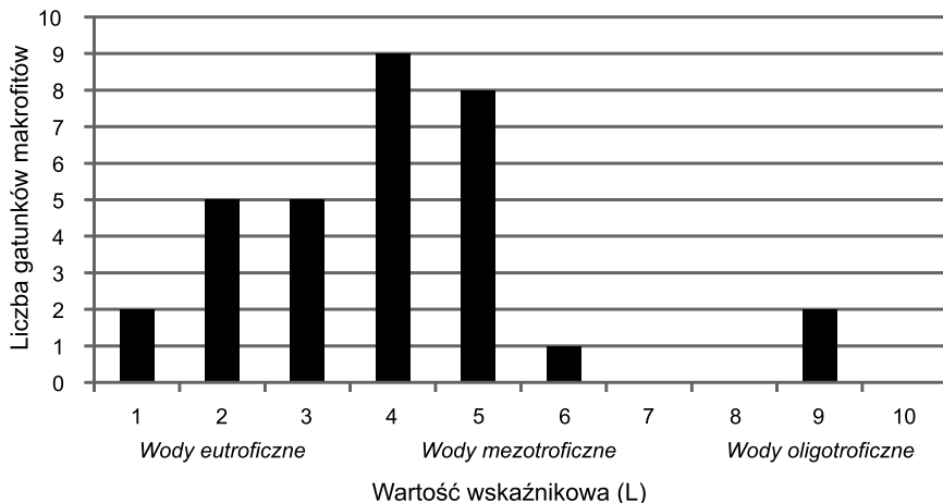
Rys. 3. Rozkład wartości wskaźnikowej ( L ) makrofitów zidentyfikowanych w trakcie badań Fig. 3. Distribution of the indicative value of species ( L ) of macrophytes identified during research
